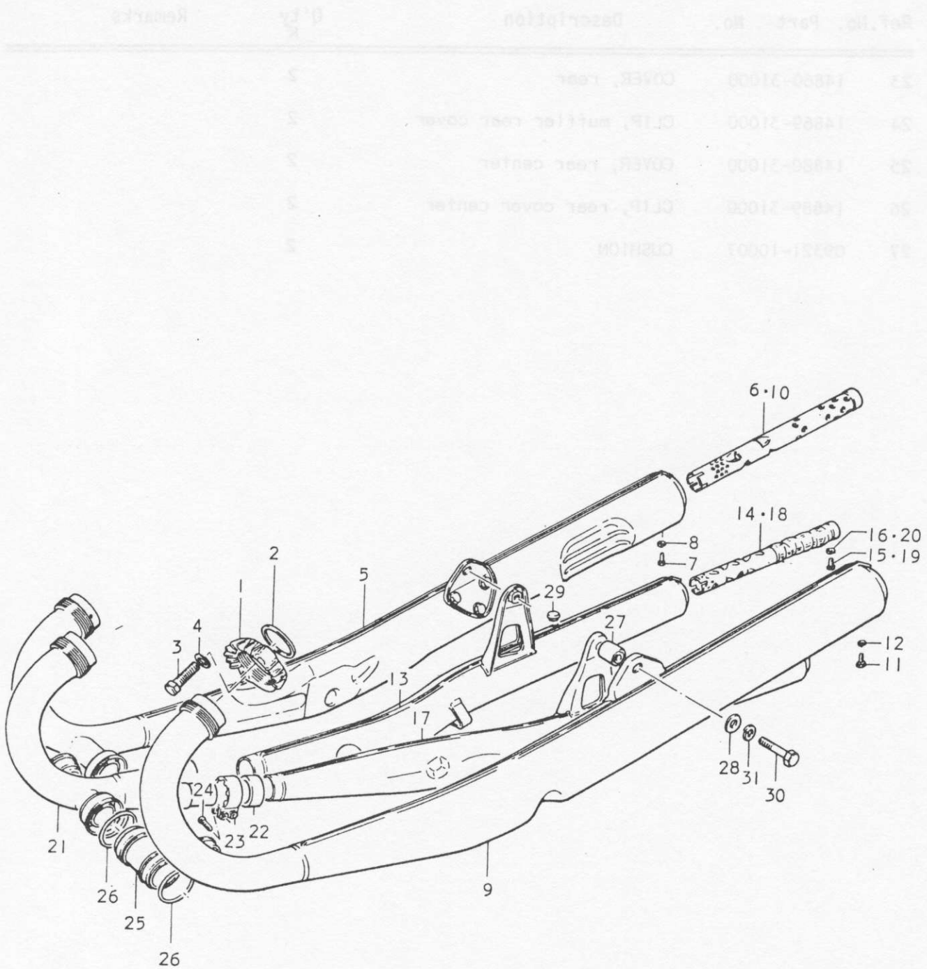
FIG. 12 MUFFLER (GT750L,M,A & B)
