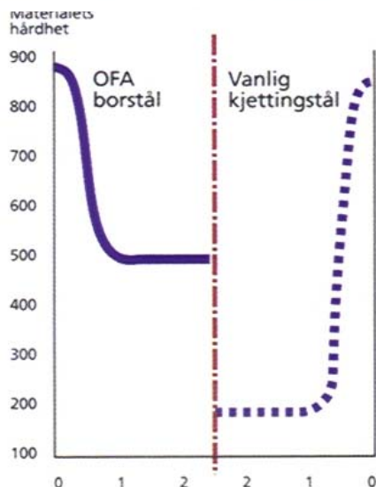
Materialhårdheten ved dybde i piggens og kjettinglenkens snittyte (Vickers-skala).
