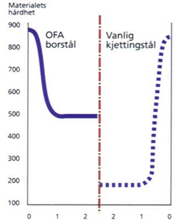
Materialhårdheten ved dybde i piggens og kjettinglenkens snitttyte (Vickers-skala).
