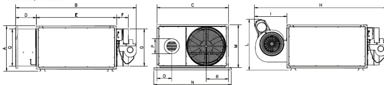
FARM150;FARM200
